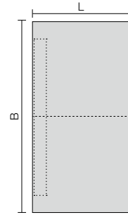
Schlüter®-KERDI-SHOWER-LTS, drenaje en el lado largo
