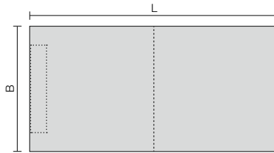
Schlüter®-KERDI-SHOWER-LTS, drenaje en el lado corto
