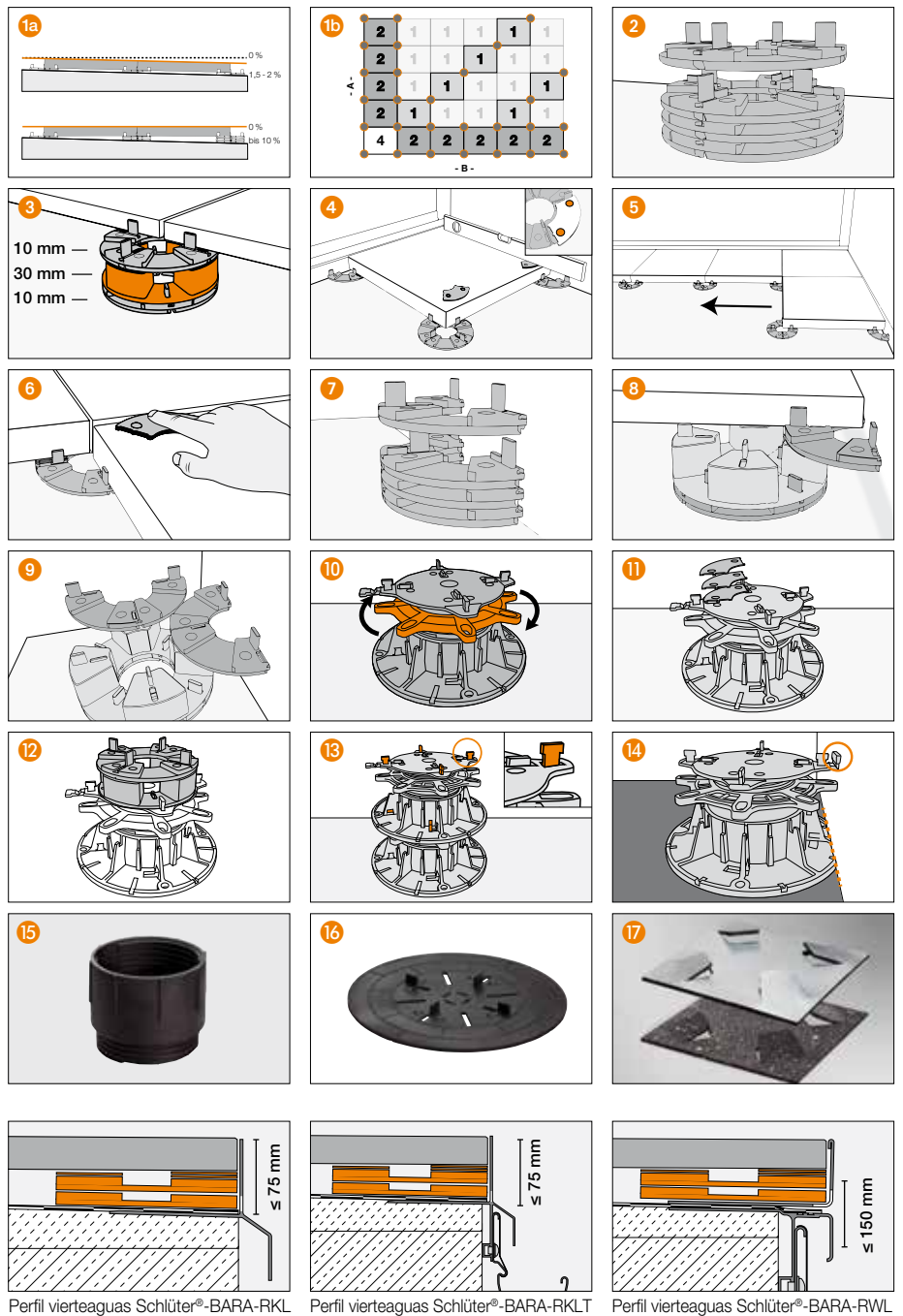
Perfil vierteaguas Schlüter®-BARA-RKL
