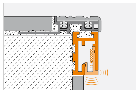
Ejemplo constructivo con el difusor Schlüter®-LIPROTEC-VBD
