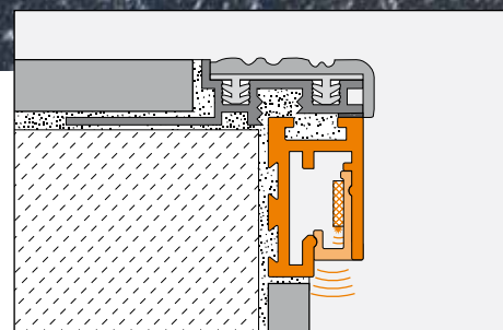
Ejemplo constructivo con el difusor Schlüter®-LIPROTEC-VBI
