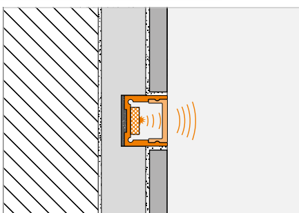
Línea de luz sobre Schlüter-KERDI-BOARD-K de 19 mm
