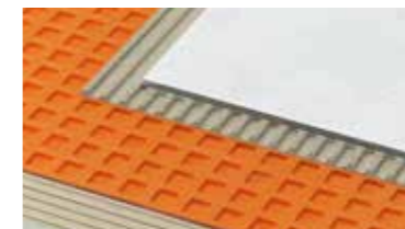
Schlüter®-DITRA 25 Lámina de impermeabilización y desolidarización para la colocación de baldosas sobre soportes críticos (p.ej. soportes de madera, yeso y soportes fisurados).
